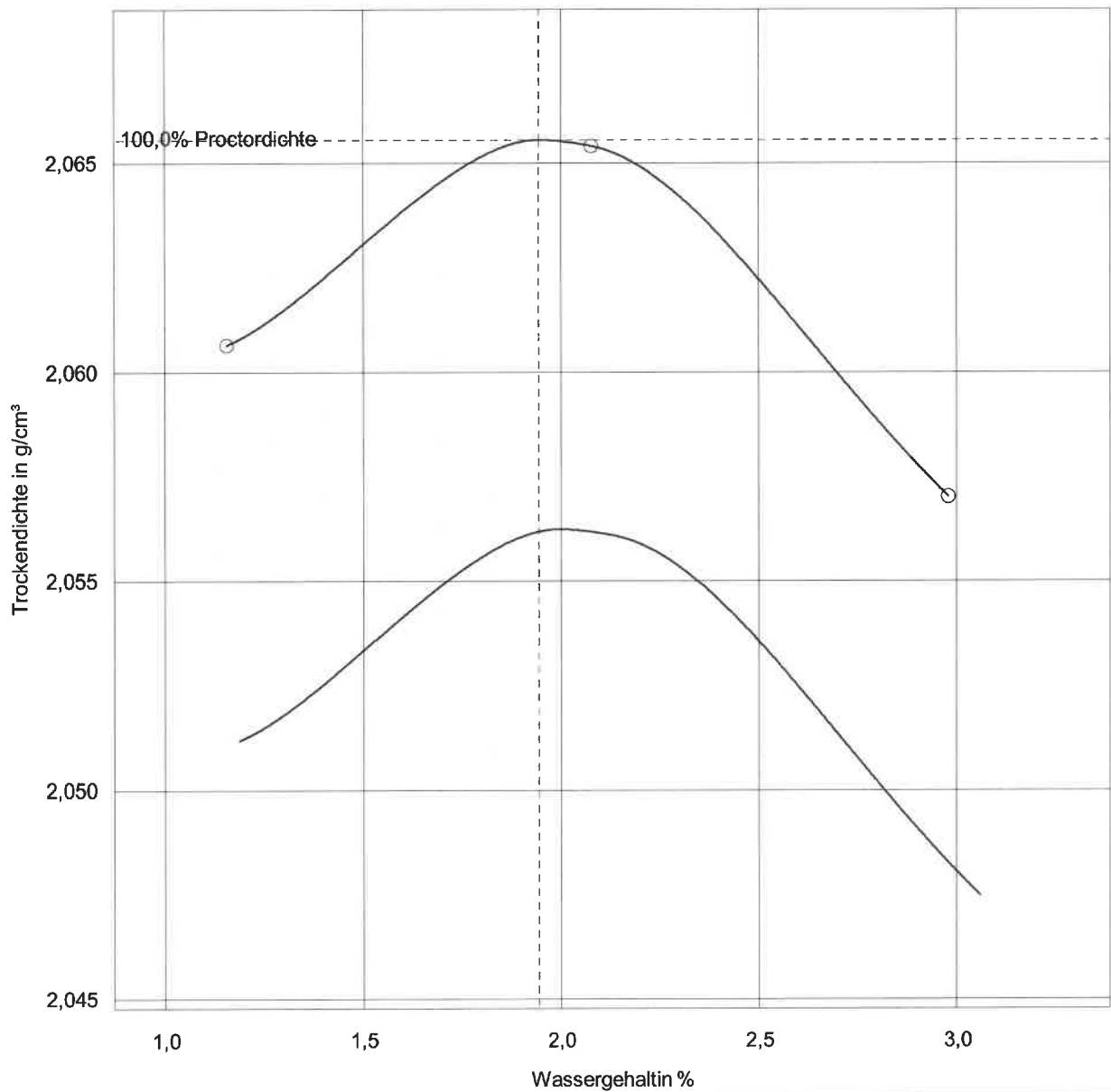
Abbildung 1: Proctorkurve korrigiert (nicht korrigiert) für Korngemisch KG 2 mit Körnung 0/32 mm
