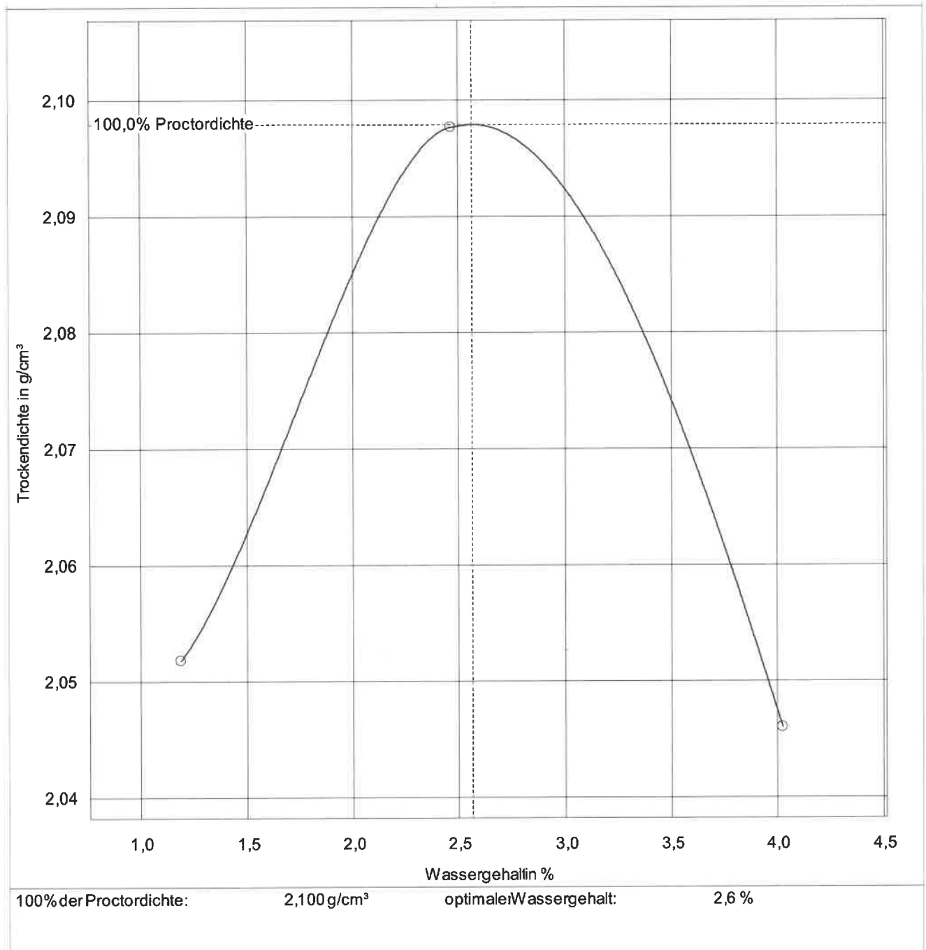
Abbildung 1: Frostschuttschicht 0/32 UF3 - Proctorkurve
