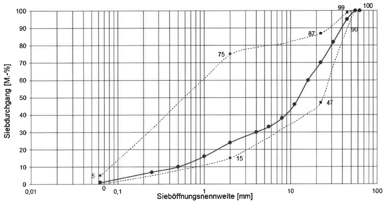
Abbildung 2: Korngrößenverteilung der Frostschuttschicht 0/45 UF 3 im Sieblinienbereich der TL SoB-StB 20
