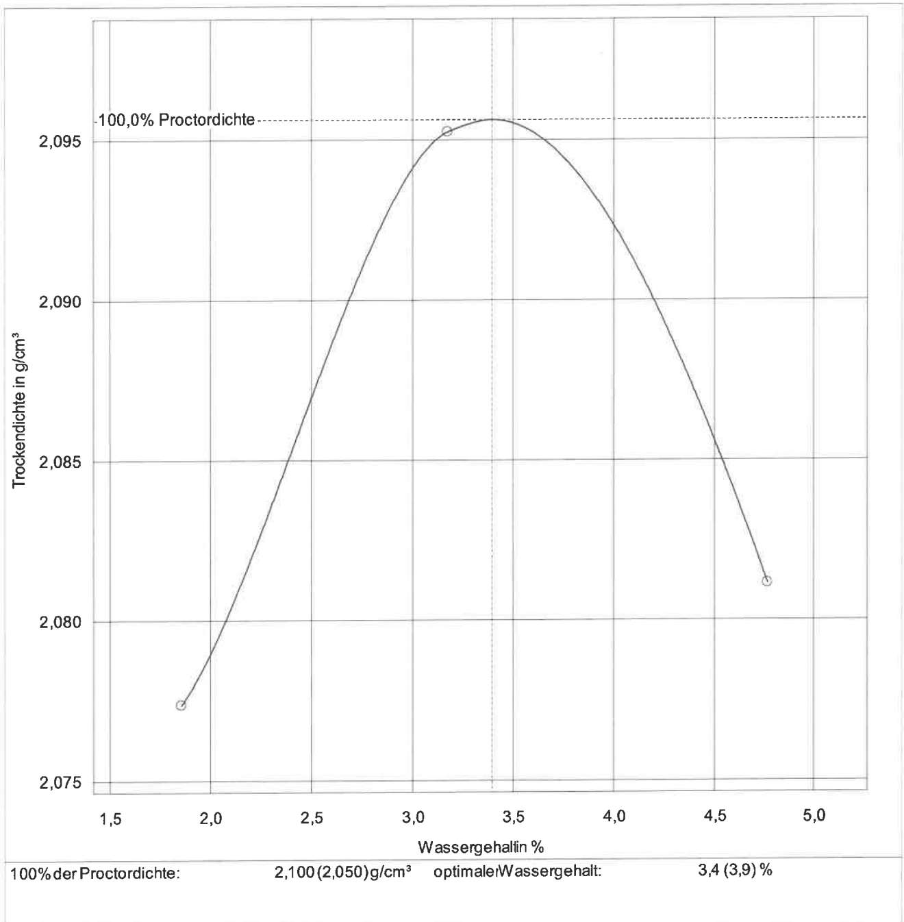
Abbildung 2: Frostschuttschicht 0/45 UF3 - Proctorkurve
