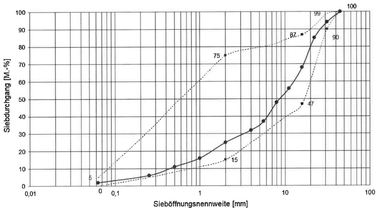
Abbildung 1: Korngrößenverteilung der Frostschuttschicht 0/32 UF 3 im Sieblinienbereich der TL SoB-StB 20
