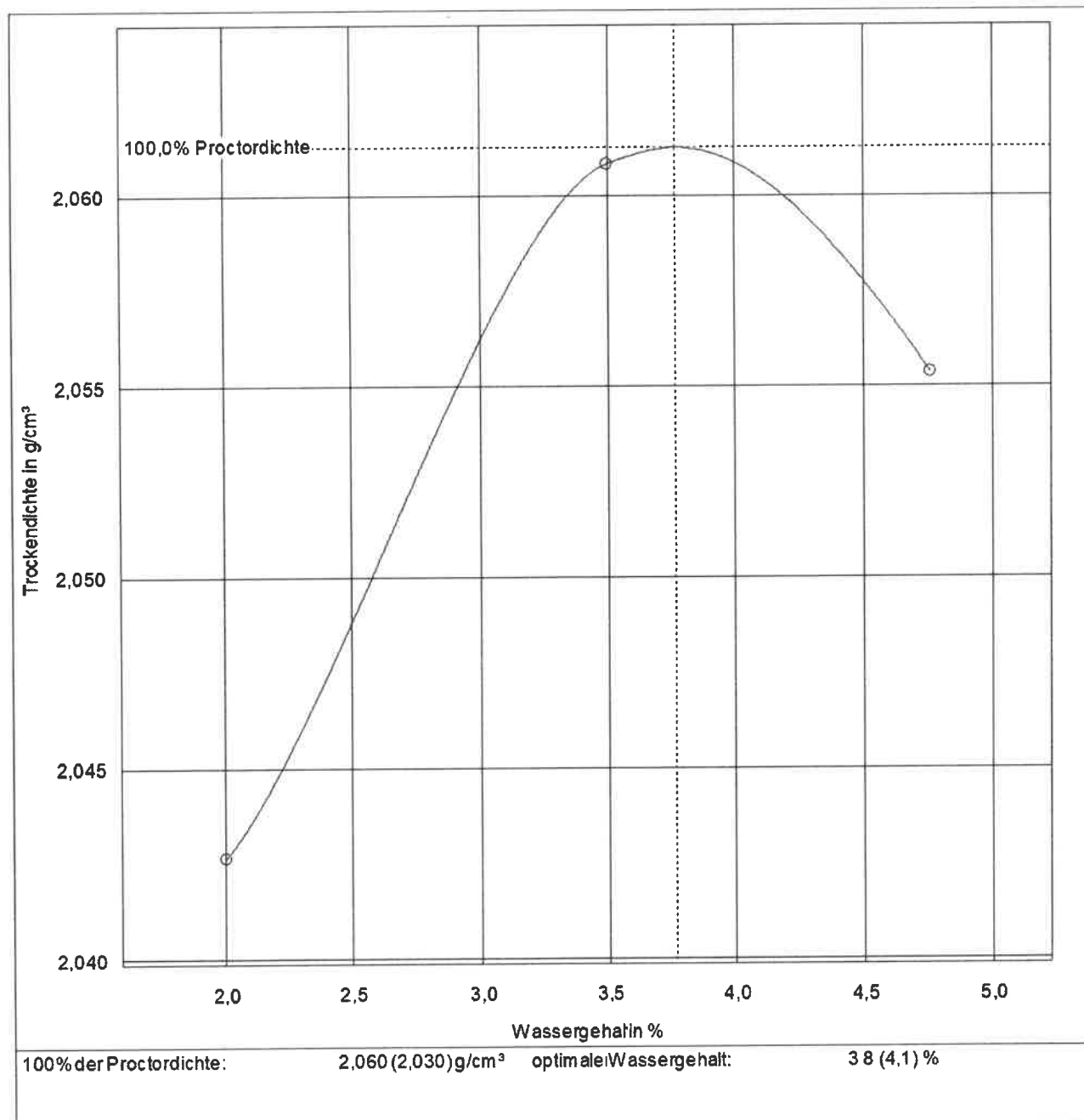
Abbildung 2: Schottertragschicht 0/45 - Proctorkurve
