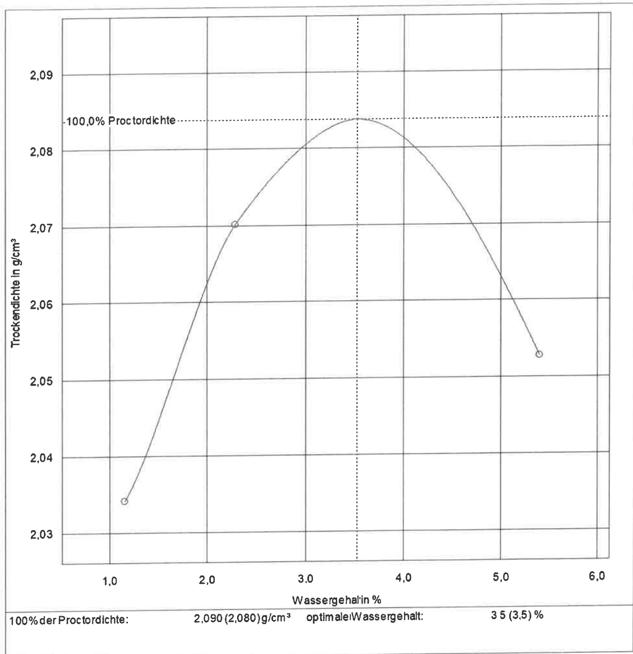
Abbildung 1: Schottertragschicht 0/32 - Proctorkurve
