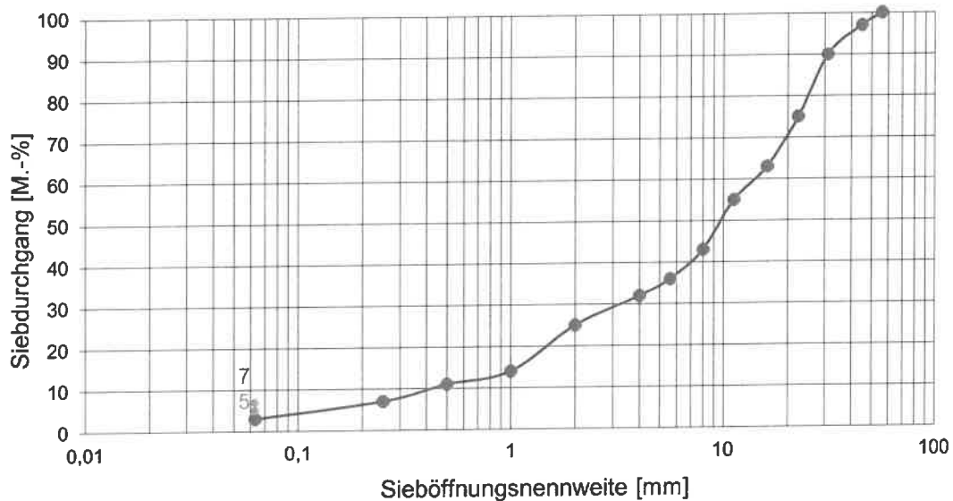
Abbildung 2: Darstellung der Korngrößenverteilung für die Tragschicht ohne Bindemittel 0/45
