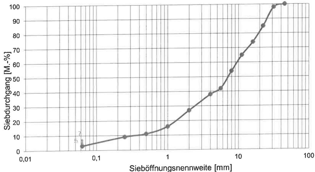
Abbildung 1: Darstellung der Korngrößenverteilung für die Tragschicht ohne Bindemittel 0/32
