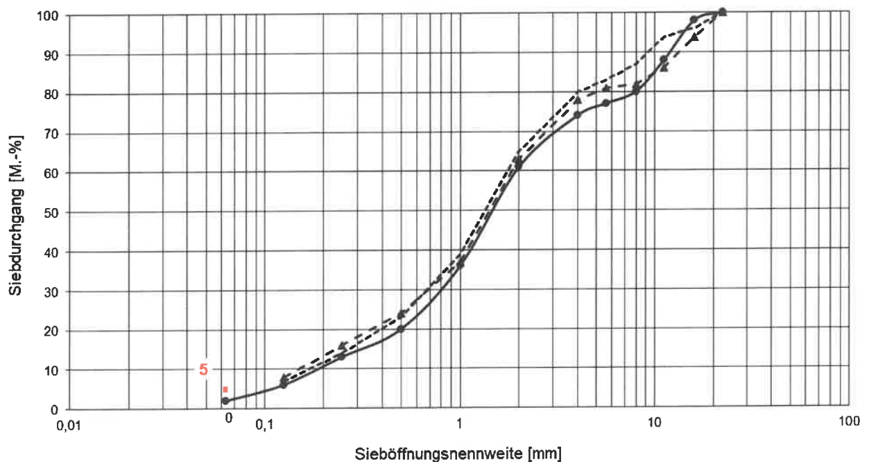
Abbildung 1: Darstellung der Korngrößenverteilung für die Dynamische Schicht 0/16 mm, durchgezogene Linie = Ausgangsmaterial, gestrichelte Linien = nach Verschleißbeanspruchung Probe 1 und Probe 2
